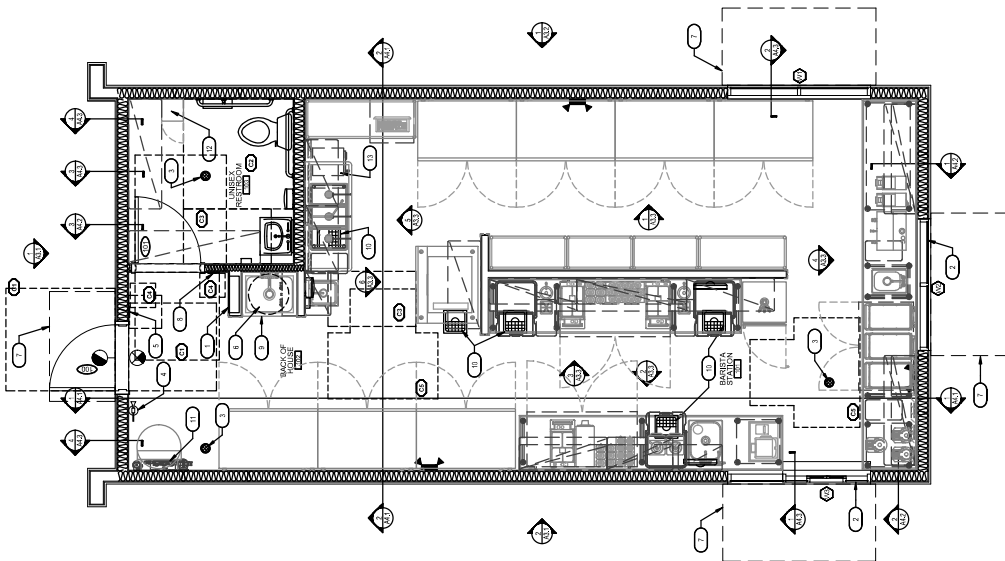
2 FLOOR PLAN SCALE: 3/8" = 1'-0"
