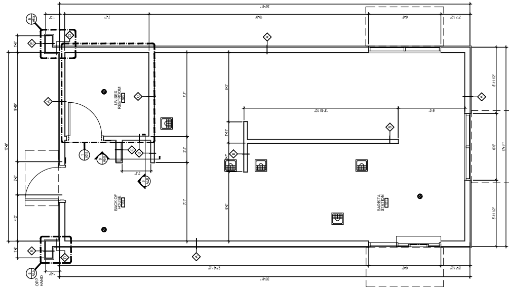
1 DIMENSION PLAN SCALE: 3/8" = 1'-0"
